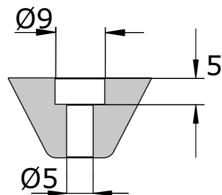
Schnittansicht A-A
