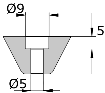
Schnittansicht A-A
